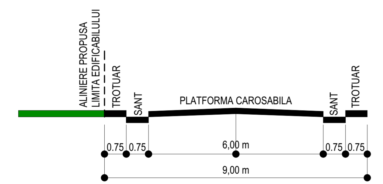
PROFIL TRANSVERSAL TIP 1 - DRUM DE EXPLOATARE EXISTENT DE 225/1 PROPUSE PENTRU MODERNIZARE
